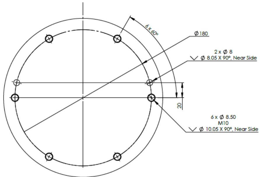
1.1: Onderkant van de basis van de robot
