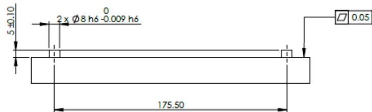
1.2: Montageplaat voor basis van de robot
