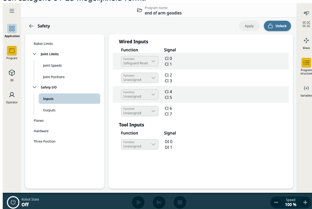
Figuur 1.4: PolyScope X-scherm met de ingangssignalen.
