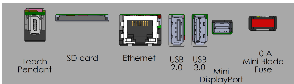
Externe aansluitpoorten.
